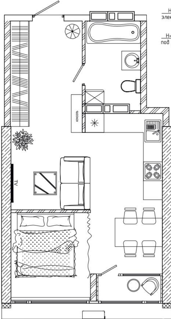
План расстановки мебели и оборудования*
