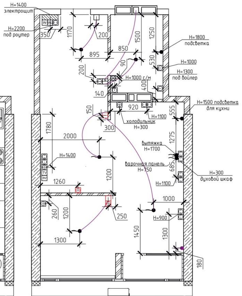
План расстановки электрооборудования
