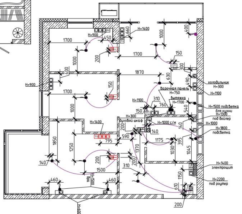
План расстановки электрооборудования
